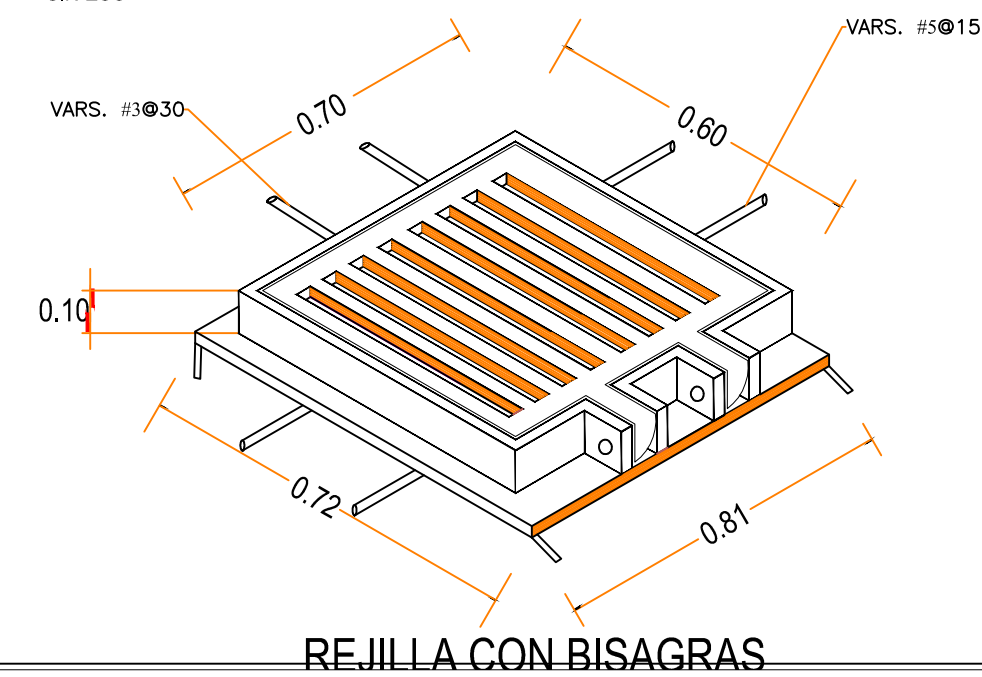
PLANTA DETALLE DE COLADERA EN VIALIDAD PUERTO
