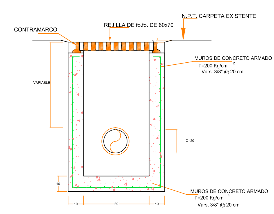
CORTE D - D'
